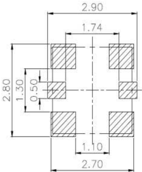
推荐的PCB布局/Recomed PCB Layout 一般公差/General Tolerance: \pm 0.05
