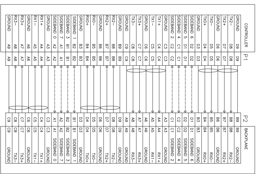
WIRING TABLE
